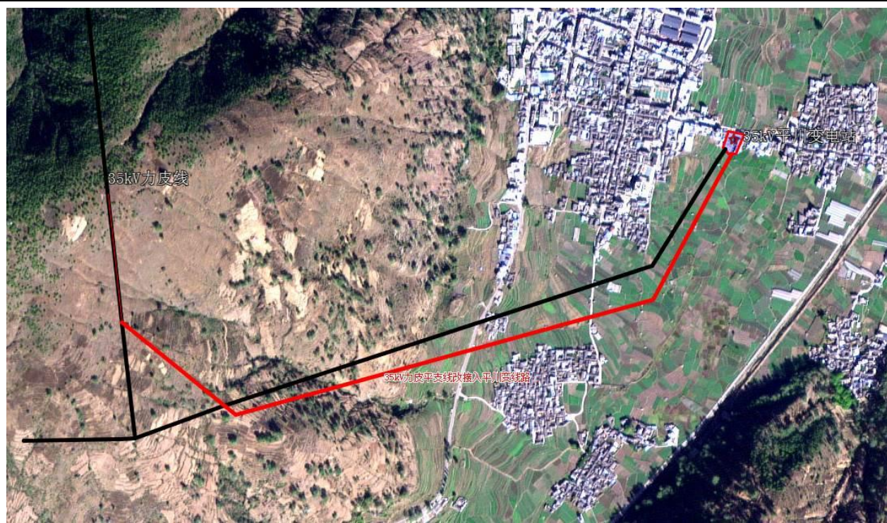
35kV 力皮平支线改接入平川变线路及变电站位置
