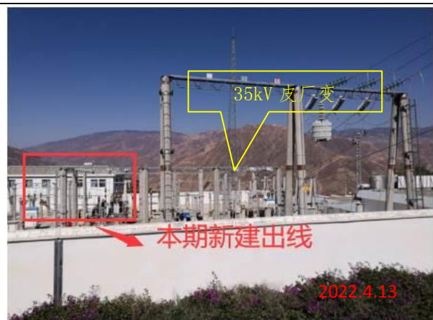
35kV 东风变~皮厂变线路
